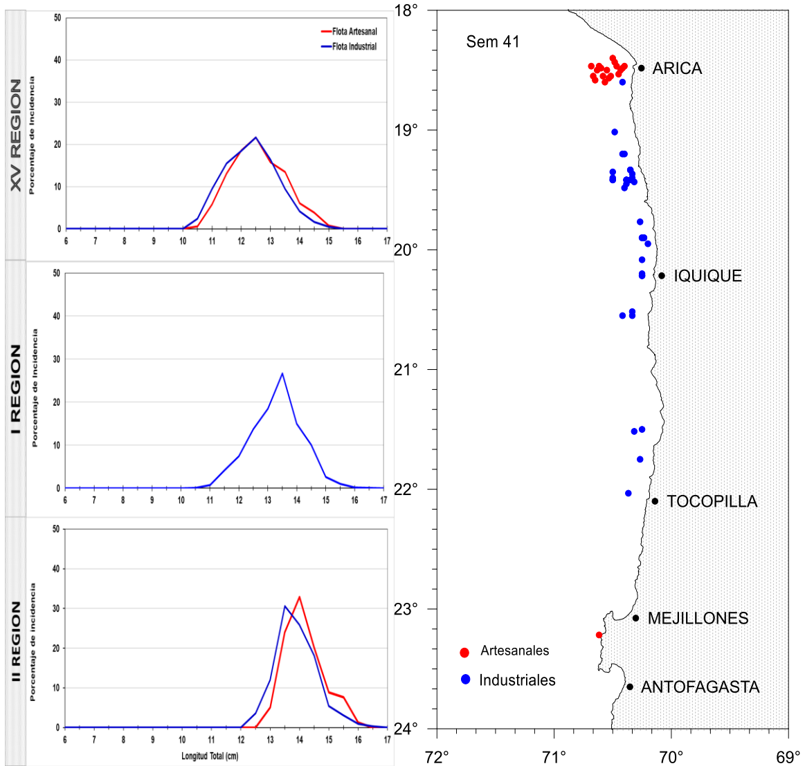
Figura 2. Estructura de talla (lado izquierdo) y posici3n geogr1fica de los viajes muestreados (lado derecho), por regi3n, correspondiente a la actividad comercial de la semana 41.
