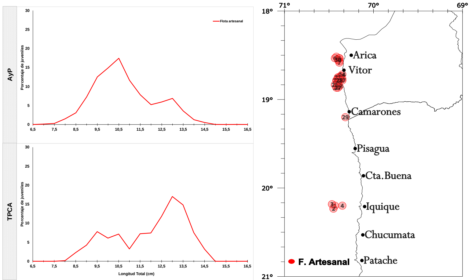
Figura 1. Estructura de talla (izquierda) y posici3n geogr3fica (derecha) de los viajes muestreados en la pesca comercial, por regi3n y tipo de flota en la zona norte.
