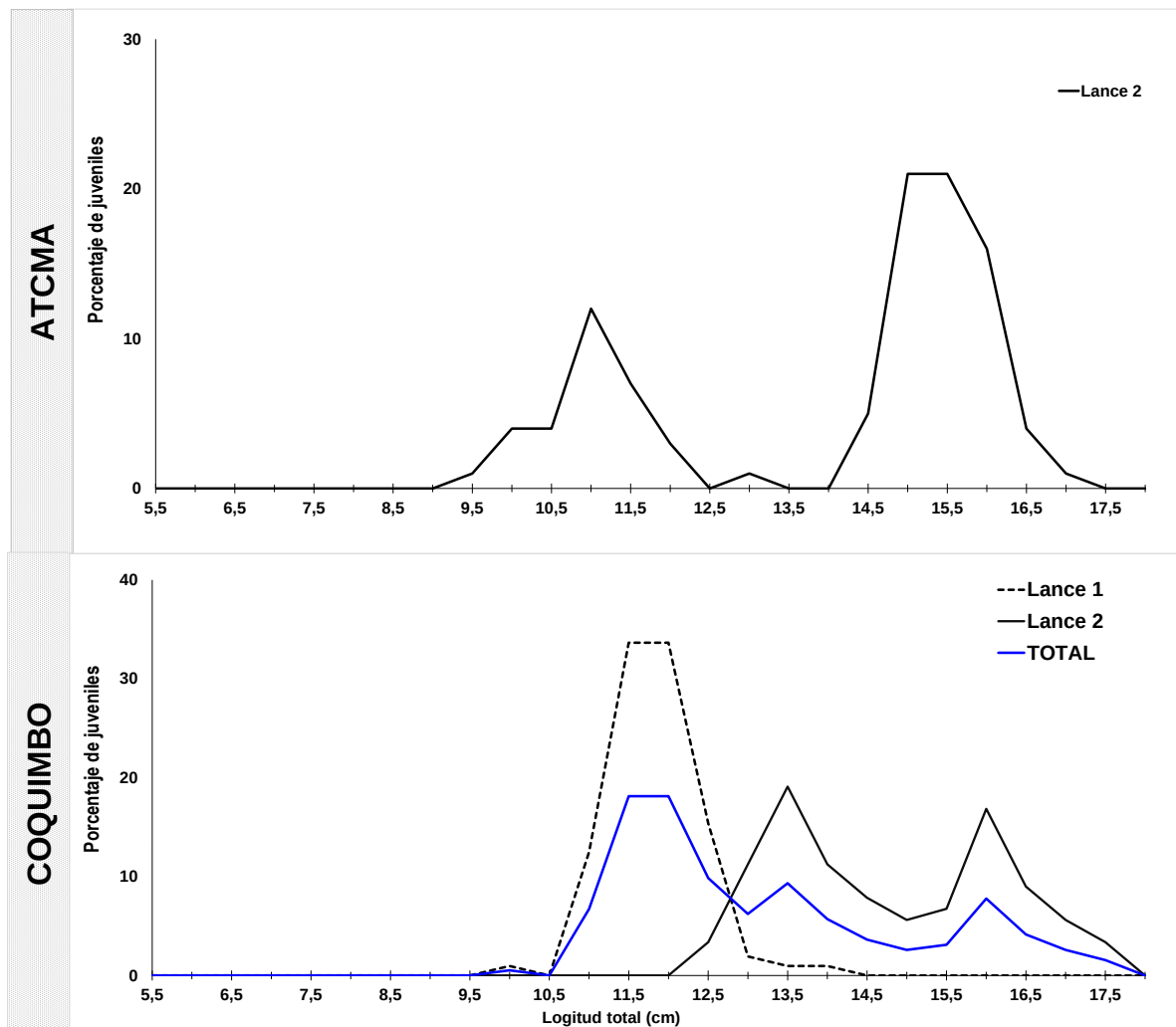
Figura 1. Estructura de talla (cm) de los lances muestreados en la PIN, zona centro norte.
