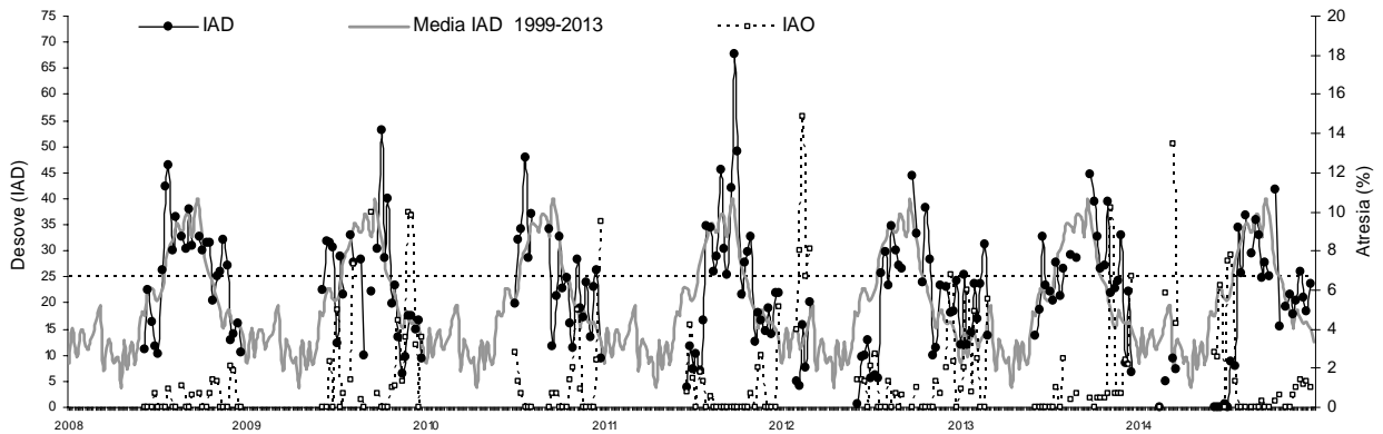
Figura 2 Comportamiento semanal del IAD e IAO en la Zona Arica – Antofagasta entre 2008 y 2014. (La lnea representa el umbral de IAD de 25% que define el periodo de los mayores desoves o de la MID).
