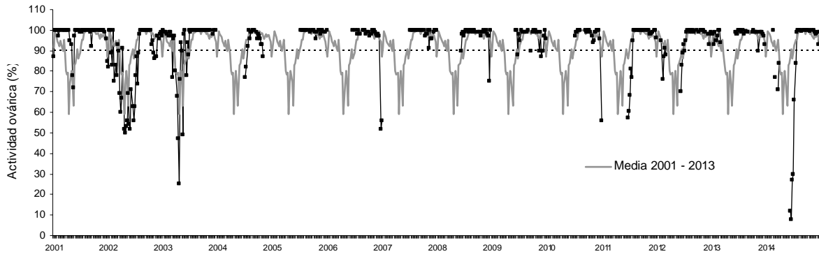
Figura 1 Incidencia semanal de hembras activas (fases agrupadas 3 a 8), aos 2001-2014.
