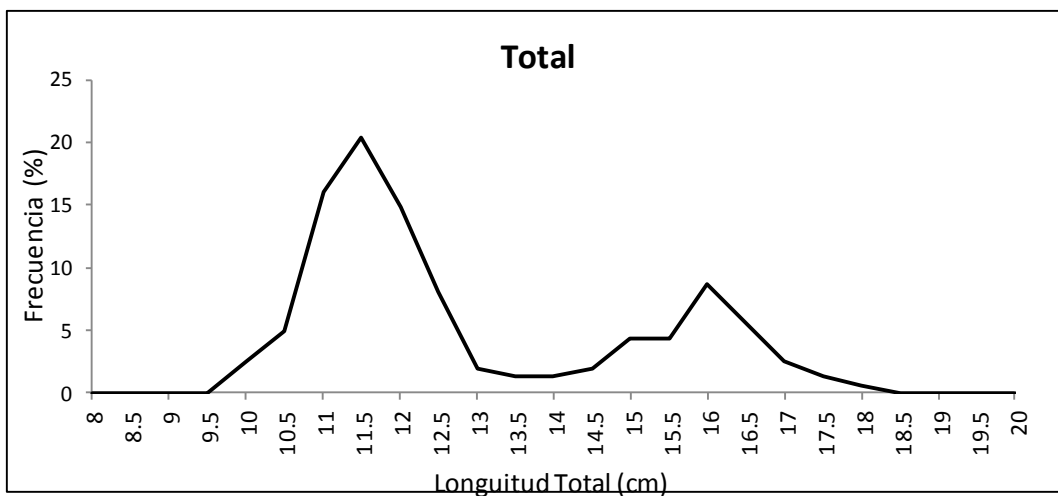
Figura 1. Distribución de tamaños de anchoveta muestreada en la Zona de Coquimbo, durante la semana 7 – 2016.
