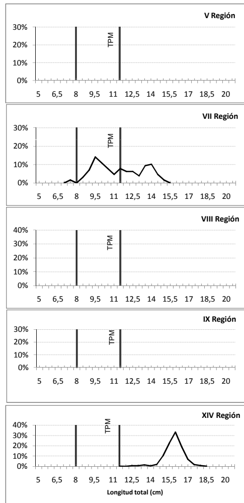
Estructura de talla de anchoveta
