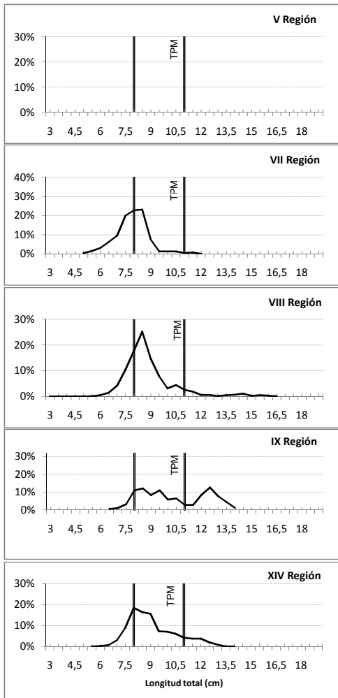
Estructura de talla de sardina común
